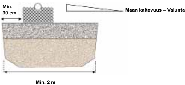
Fig. 3 Siltti, moreeni
